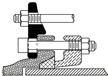
TYPE D'INSTALLATION SDR 26
