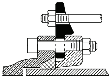
TYPE D'INSTALLATION C900 OU DR 18
